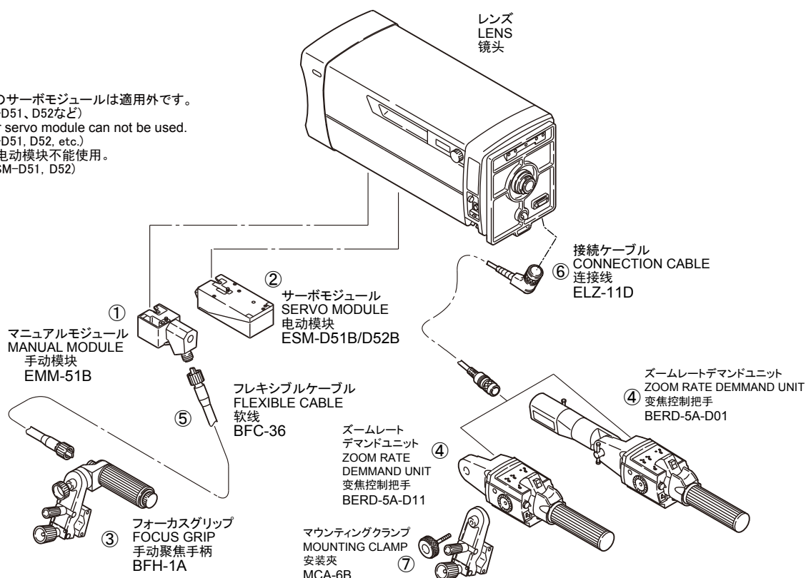
システム図 (例) Configuration (Ex.) 配置图 (例)
