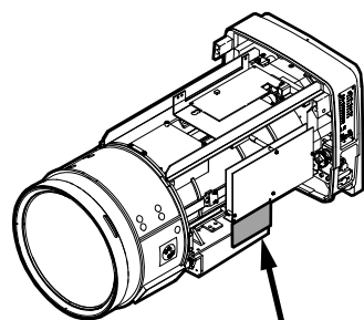
F-ボード F-BOARD F-电路器
